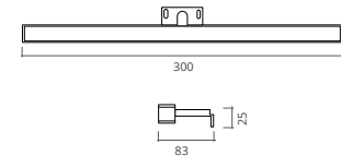
VEGA APLIQUE LED CROMADO COM MULTIGANCHO
