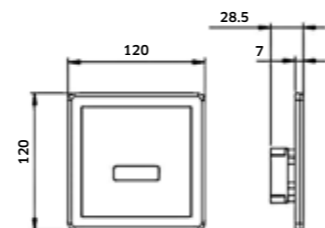
Torneira de Sensor de Lavatório 1 Água (4AA 6V/220V)
