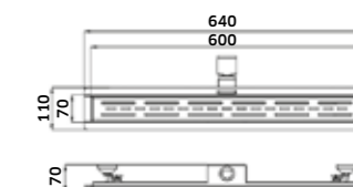
Canelete de Duche Horizontal c/ Grelha Perfurada Inox 700mm
