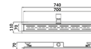
Canelete de Duche Horizontal c/ Grelha Perfurada Inox 800mm
