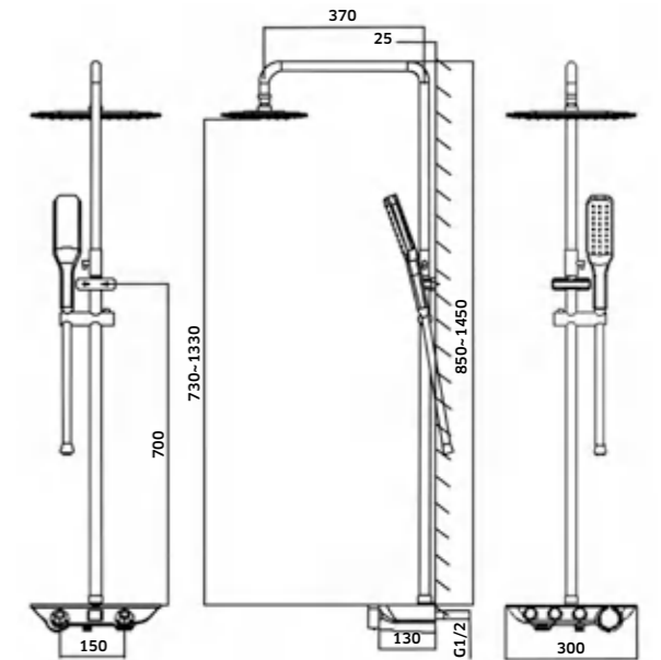
Coluna de Chuveiro c/ Torneira Monocomando LINEA
