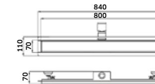
Canelete de Duche Horizontal Grelha Invertida Inox 900mm
