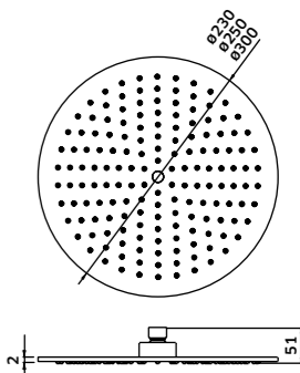
Chuveiro de Teto Redondo Ø300x2 mm
