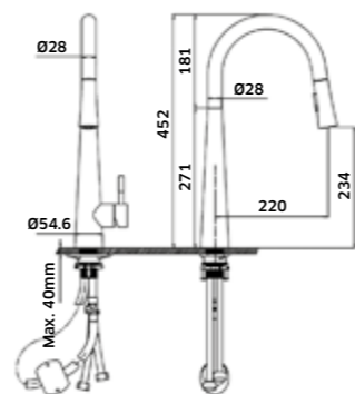
Monocomando de Banca c/ Chuveiro Extensível LAGOS
