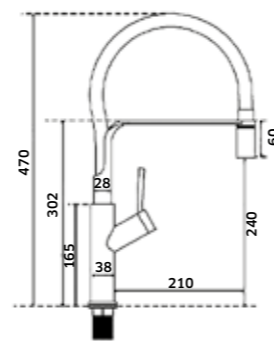
Monocomando de Banca c/ Chuveiro Extensível MILLENIUM
