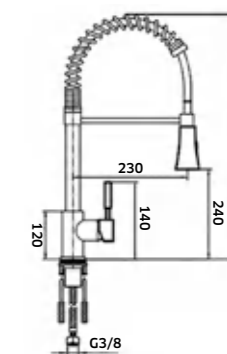
Monocomando de Banca c/ Mola e Chuveiro Extensível DOMUS
