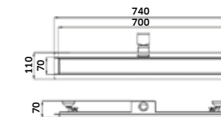
Canelete de Duche c/ Sifão Rotativo 360° Inox 800mm
