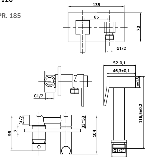
Monocomando de Encastrar Sanita/Bidé c/ Chuveiro Latão FOCUS
