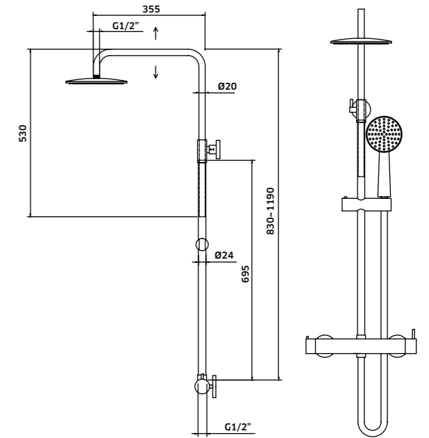
Coluna de Chuveiro c/ Torneira Monocomando FOZ
