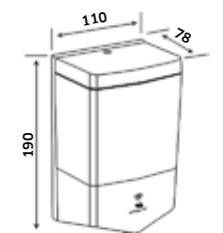
Dispensador de Toalhas de Papel Capacidade p/ 200 Folhas ■ Inox Satinado REF. DIO200. 59 ■ Preto Mate REF. DIO200PR. 75
