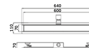
Canelete de Duche Horizontal Grelha Invertida Inox 700mm
